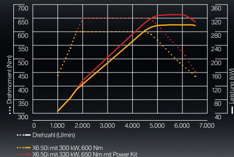
Leistungswerte des BMW X6 50i mit BMW Performance Power Kit
